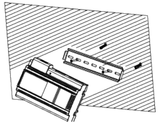
Abb. 11: Montage Versorgungs- und Steuergerät
