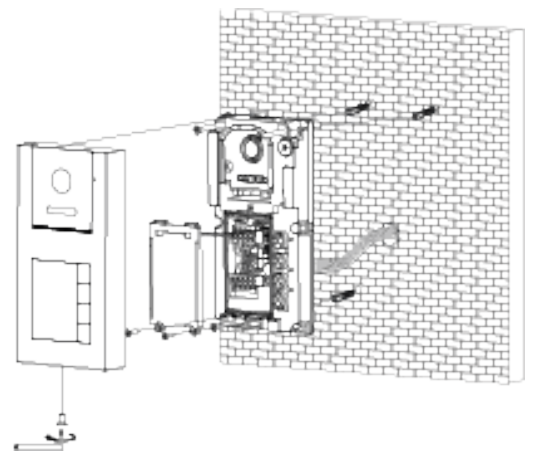
Abb. 6: Wandmontage Video-Außenstation
