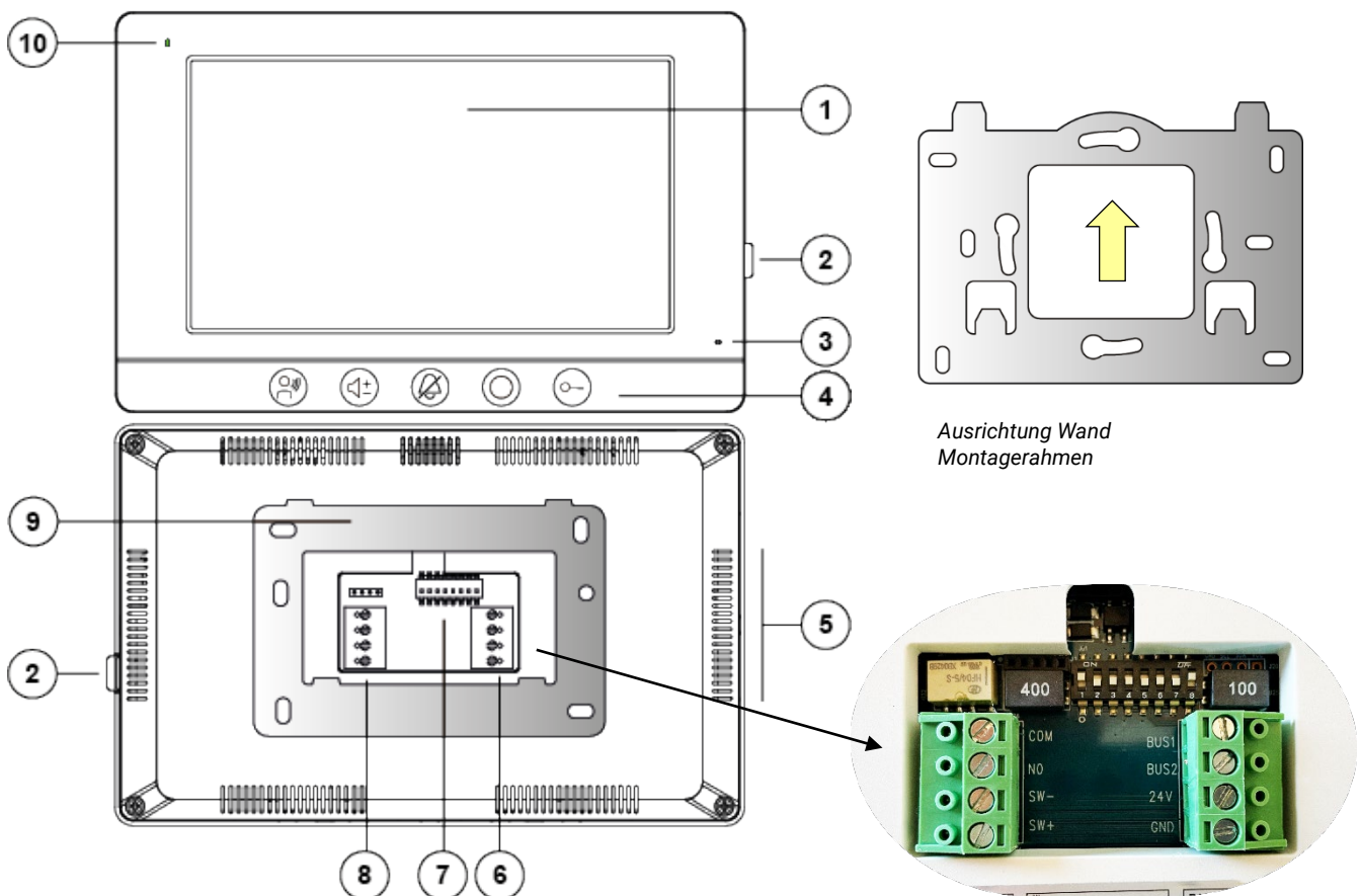
Abb. 2: Geräteübersicht Video-Innenstation
