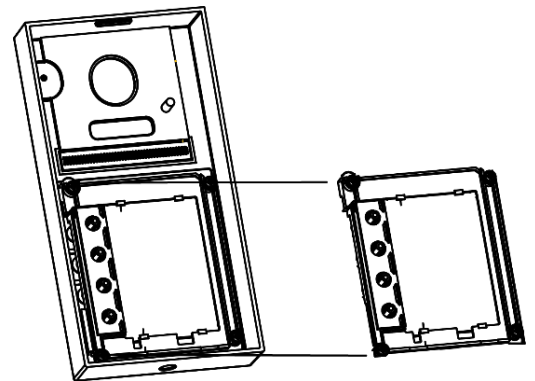
Abb. 14: Tastenmodul im Gehäuseoberteil austauschen
