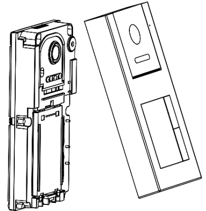
Abb. 13: Video-Außenstation öffnen
