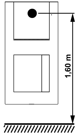
Abb. 4: Montagehöhe Video-Außenstation
