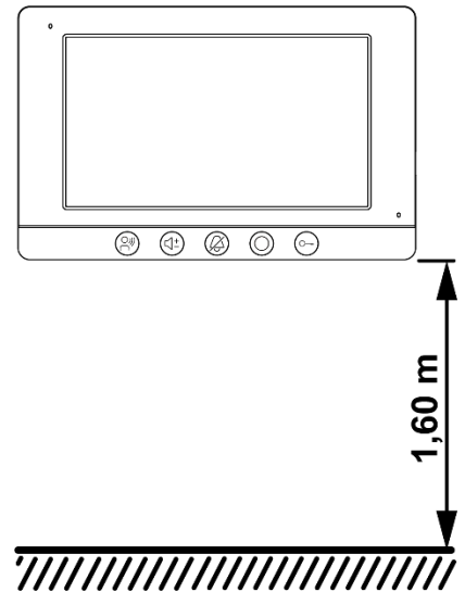
Abb. 8: Montagehöhe Video-Innenstation
